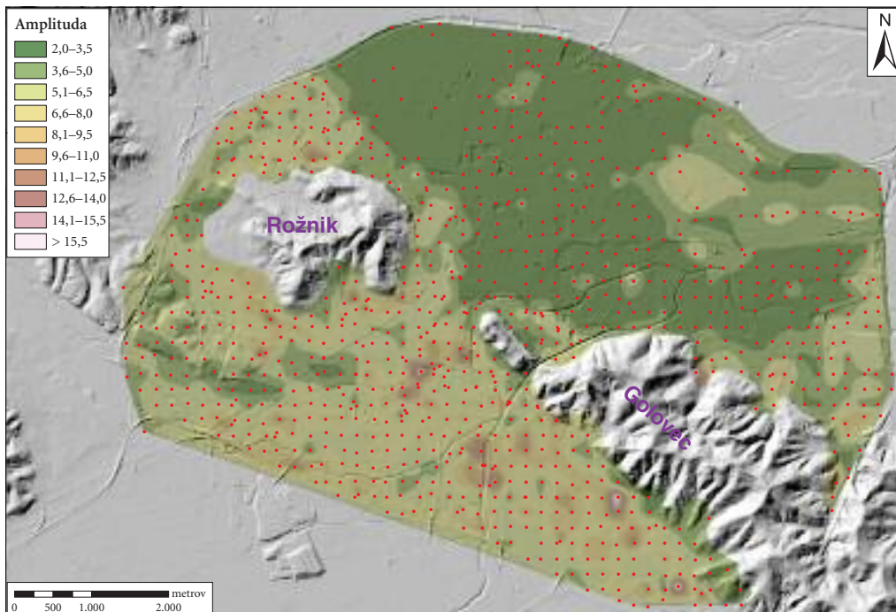
Slika 6: Karta amplitud vrhov HVSr krivulj.
