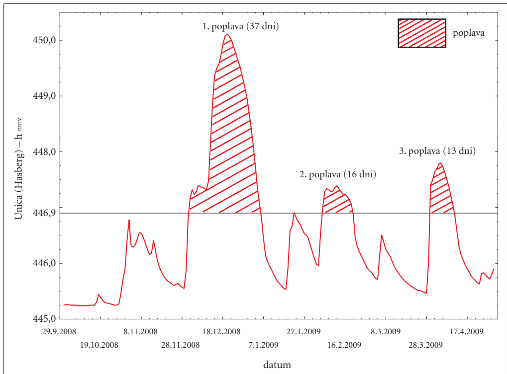
Slika 4: Poplave na Planinskem polju v obdobju 1. 10. 2008–30. 4. 2009.
