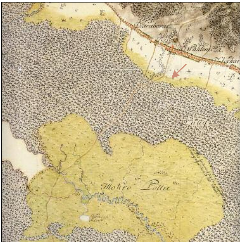
Slika 1: Lega naselij in potek prometnice sta se prilagodila nižinskim poplavam, kot kaže primer iz Slavonije na Jožefinskem vojaškem zemljevidu iz konca 18. stoletja (Zorn 2007, 131). Puščica kaže obseg vsakoletnih poplav.
