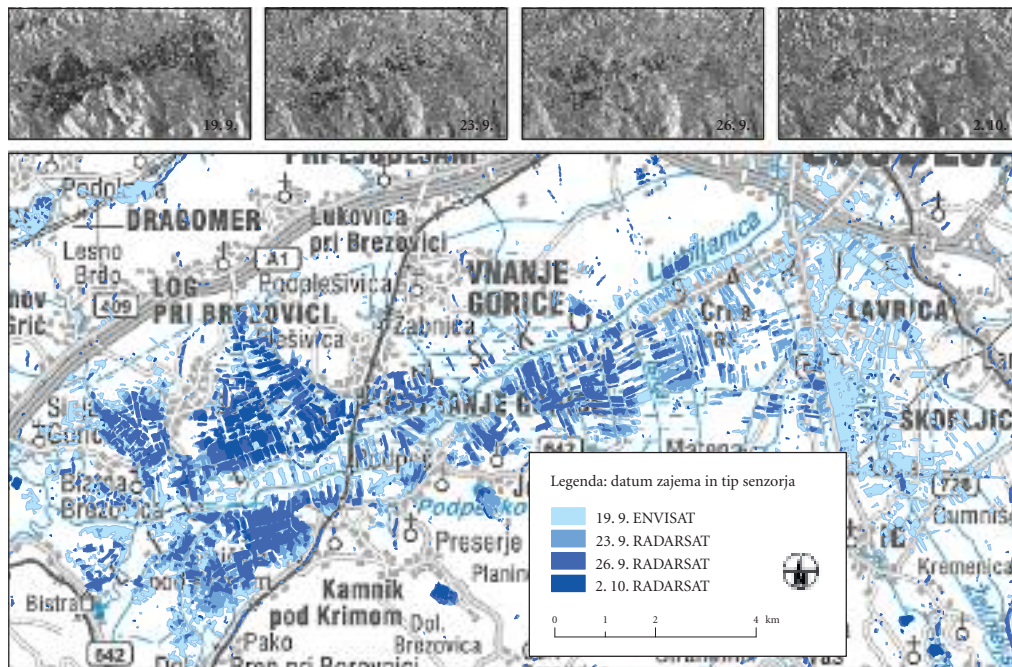
Slika 3: Zgoraj: izdelki radarskih posnetkov za izbrane datume opazovanja poplav na Ljubljanskem barju. Spodaj: dinamika poplavljenosti na Ljubljanskem barju, zaznana iz radarskih posnetkov 12,5-metrске ločljivosti, zajetih 19. 9., 23. 9., 26. 9. in 2. 10. 2010.
