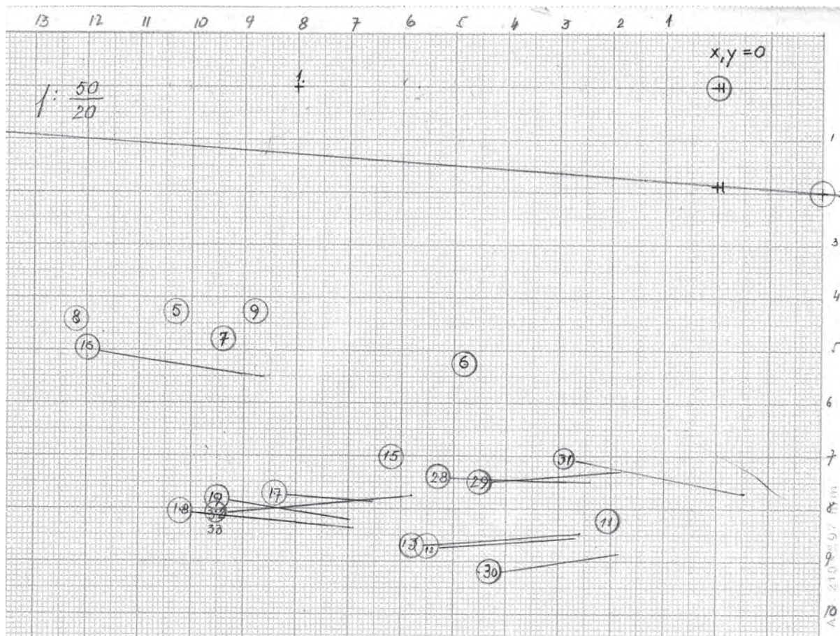
Bercetov tloris dela grobišča, M. = 1 : 20 (hrani NMS, AO, arhiv št. 435)
