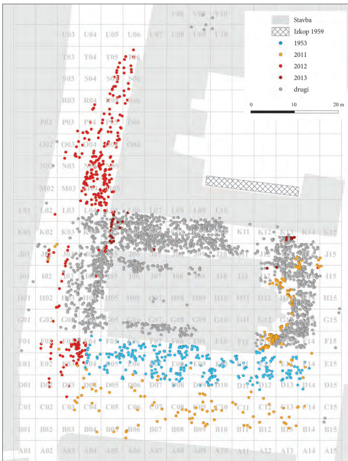
Sl. 2: Načrt grobišča z izpostavljenimi grobovi, izkopanimi leta 1953 in 2011–2013.
