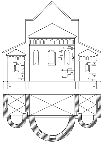
Apsida
