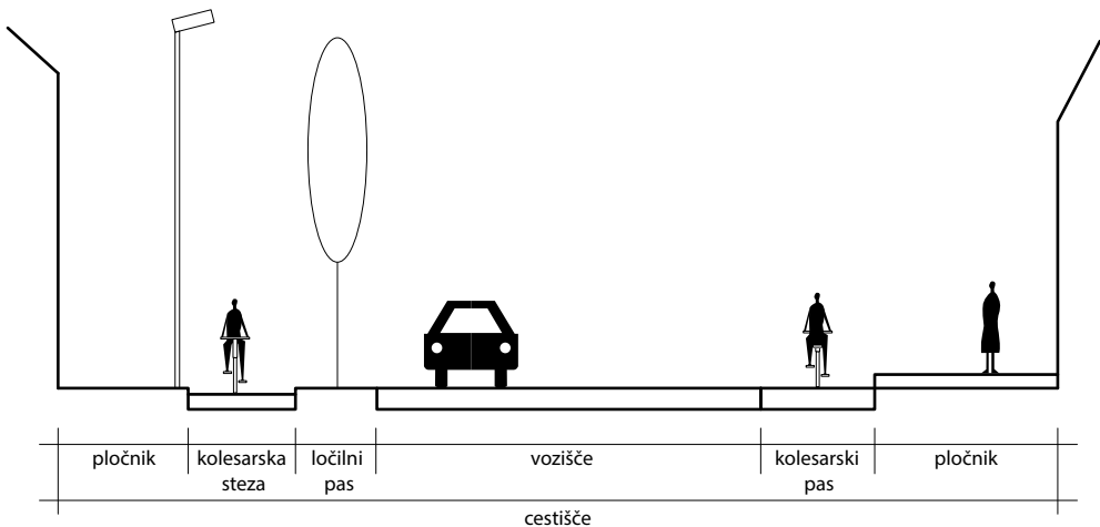
PREČNI PREREZ ULICE
