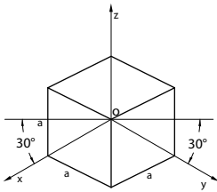
izometrija
