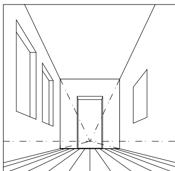
Žabja perspektiva
