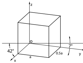
dimetrija
