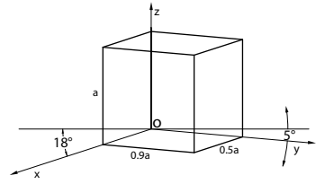
trimetrija
