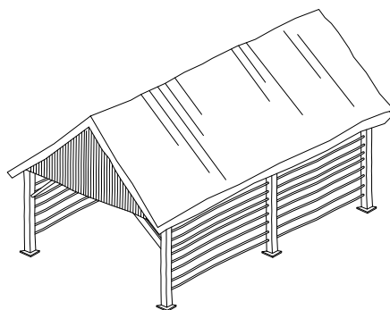
Dvojni kozolec
