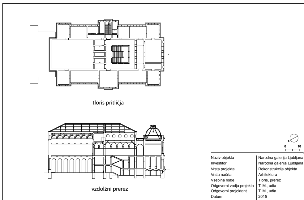
Arhitekturni načrt za rekonstrukcijo Narodne galerije v Ljubljani
