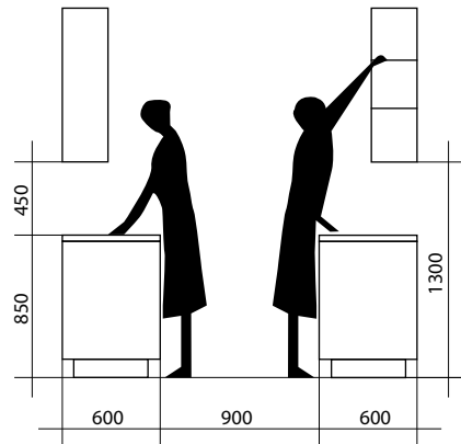
Dimenzioniranje notranje opreme v človeškem merilu
