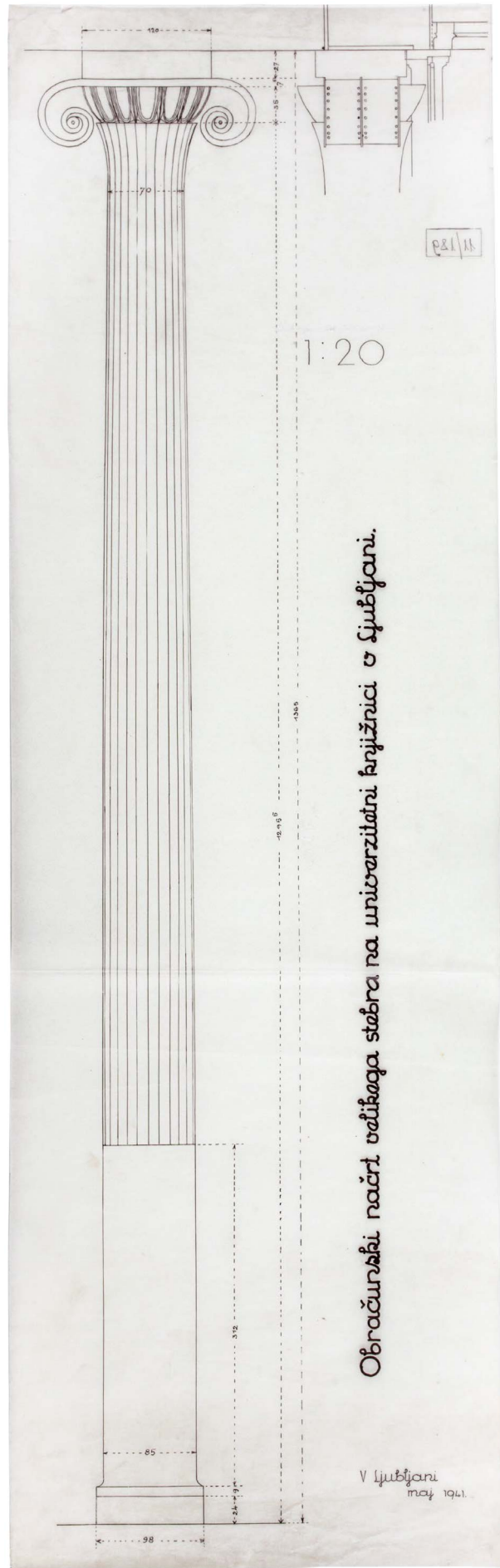
XLI - Steber pred čitalniškim oknom, obračunski list, 1:20, 5. 1941
