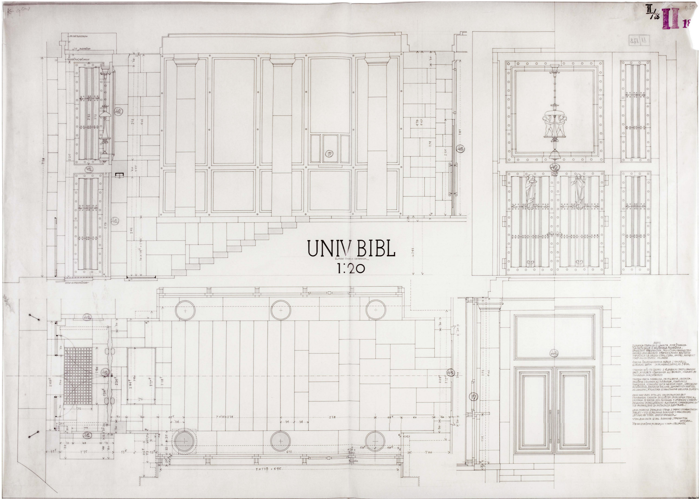
LIV - Načrt glavnega vhoda z vežo, 1:20, 20. 1. 1938
