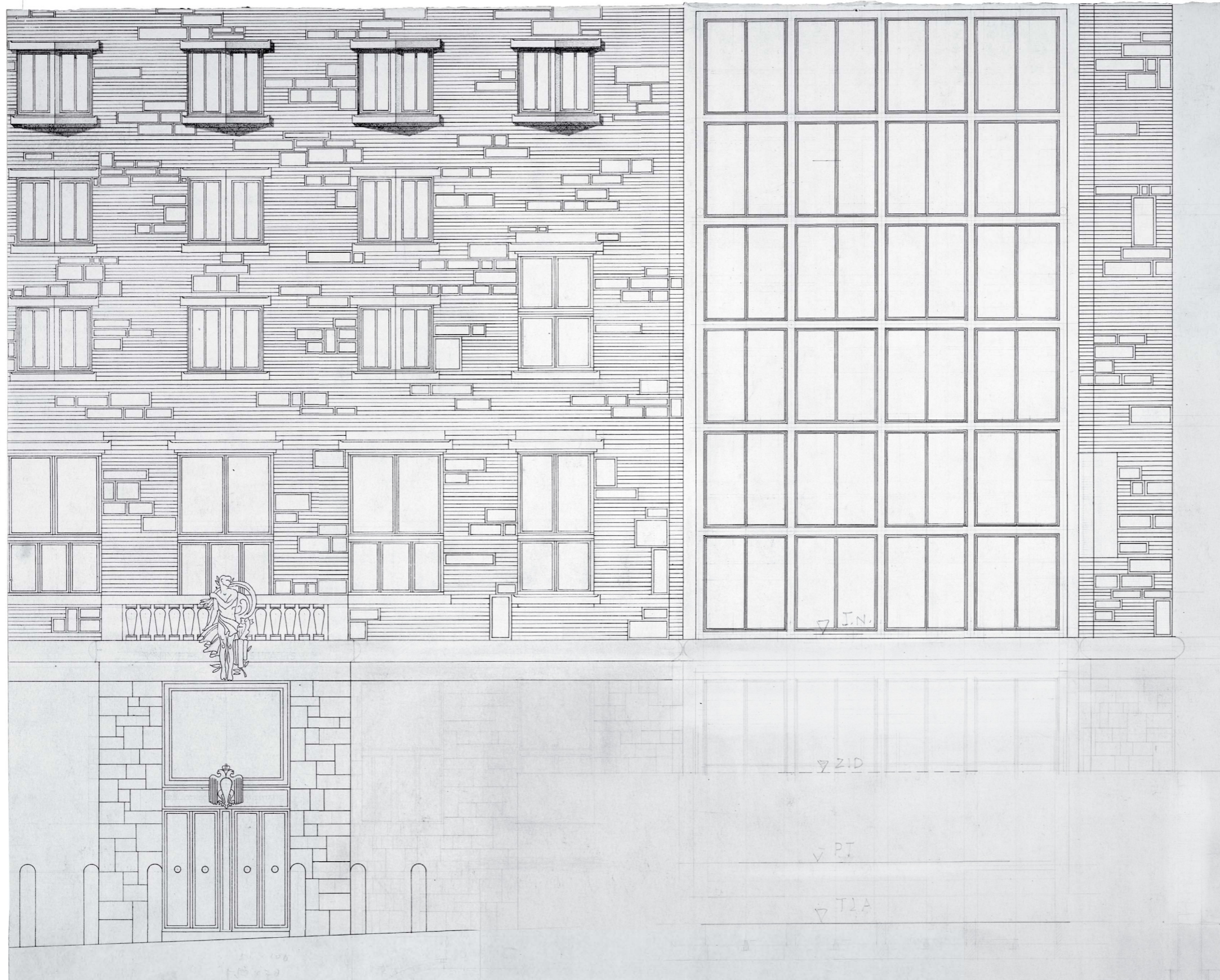
XXVIII - Del vhodne fasade s čitalniškim oknom na Vegovo ulico, 1:100, 1936
