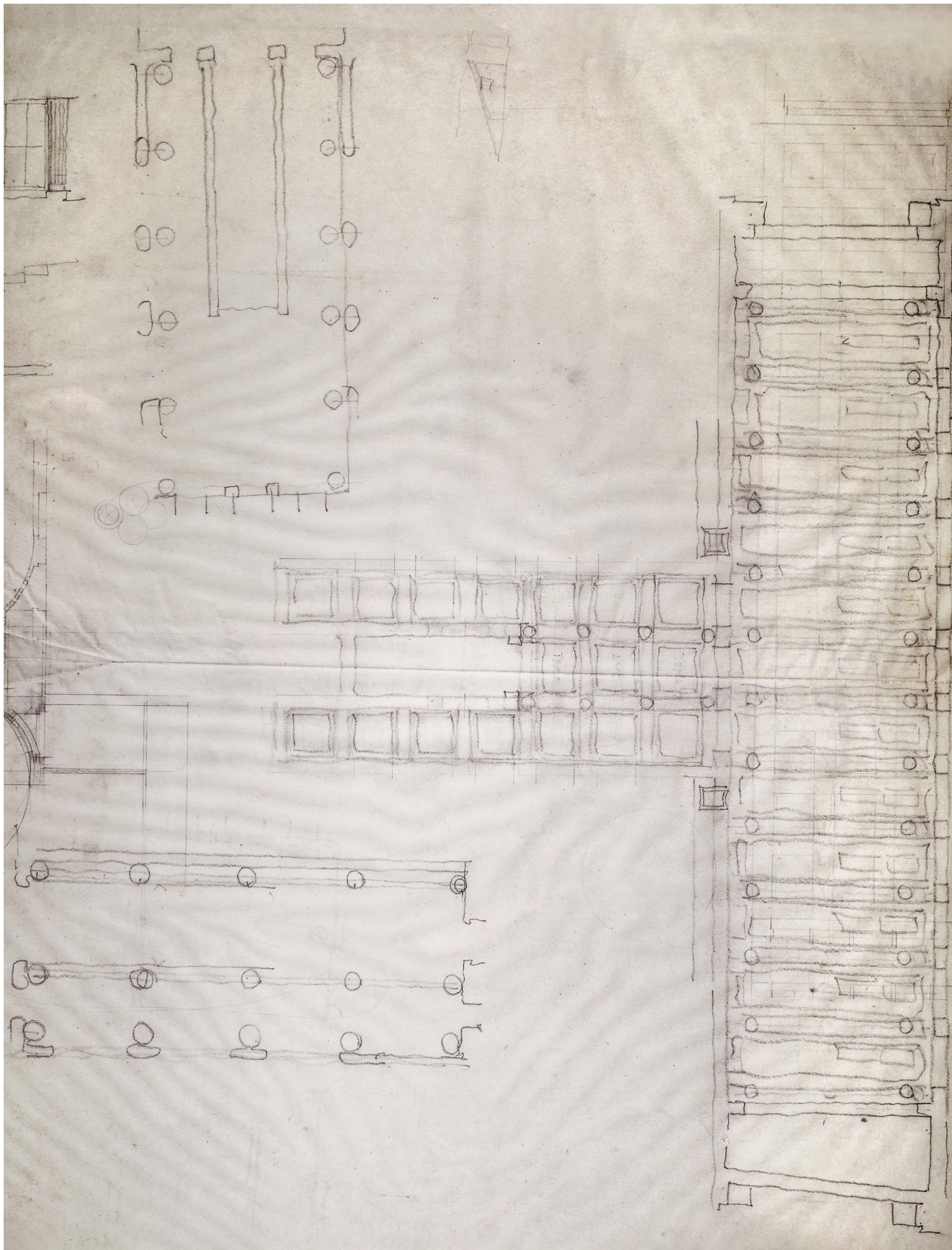
LXX - Plečnikova skica peristila s čitalnico,
