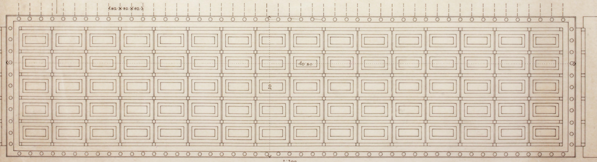
LXXVIII - Načrt čitalniškega stropa, 1:20
