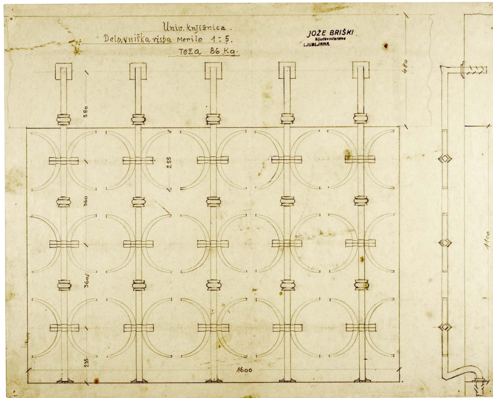
XXXVI-XXXVII - Skici okrasnih mrež kletnega okna na Gosposki ulici, 1940
