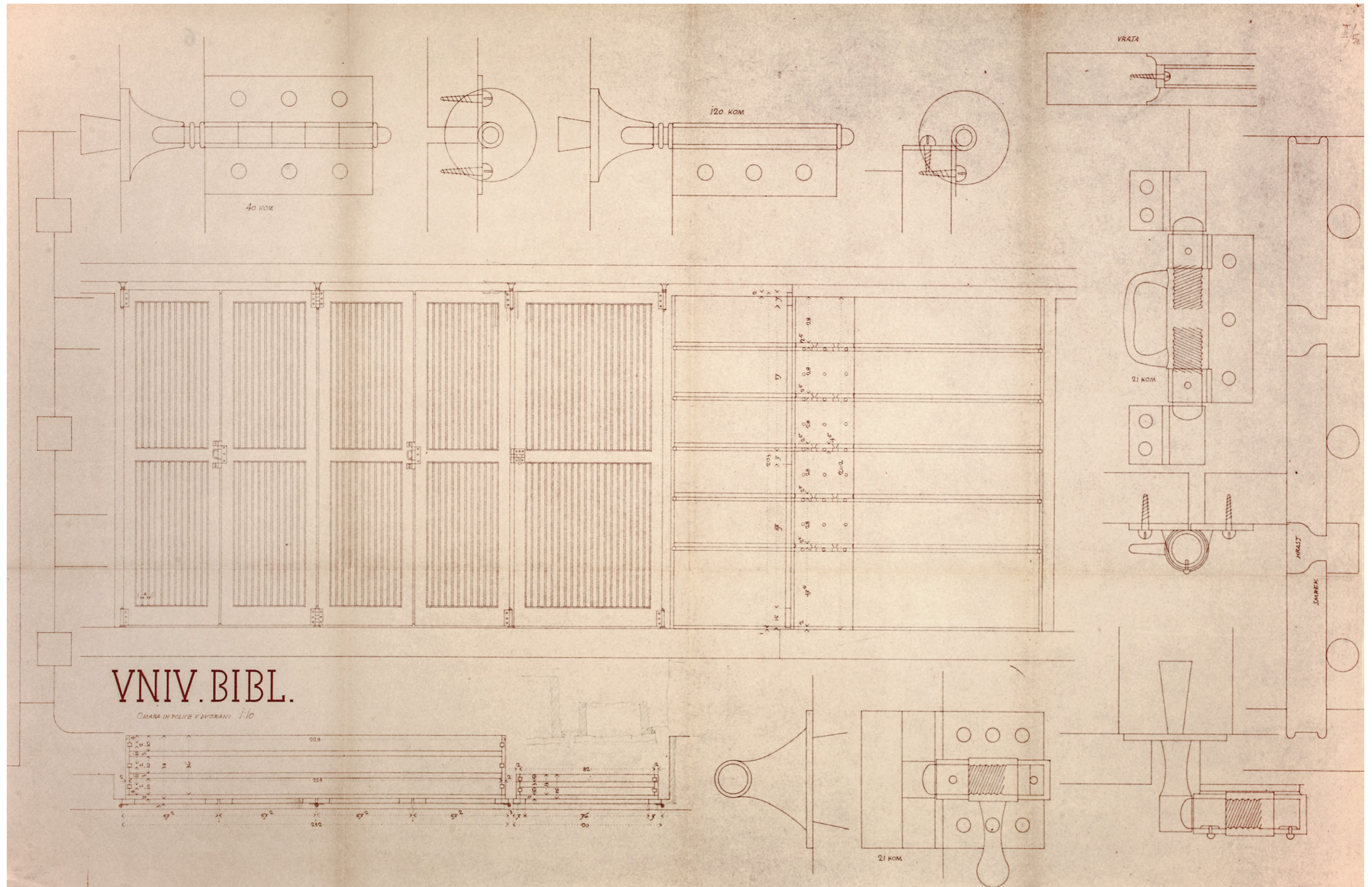
LXXXVIII - Načrt omar in polic v čitalnici, 1:10, 8. 1940
