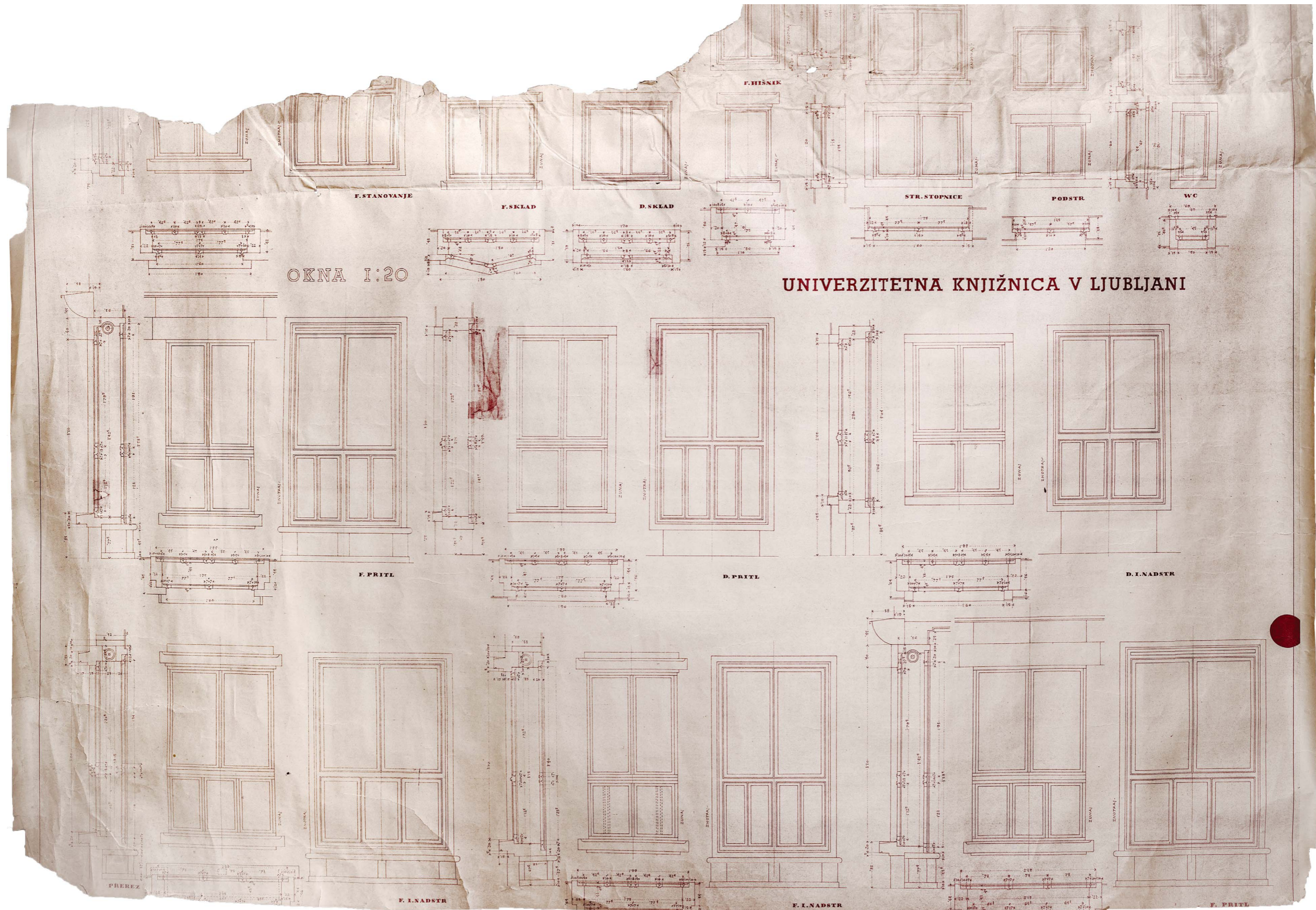
LIII - Načrt oken, ozalidna kopija, 1:20
