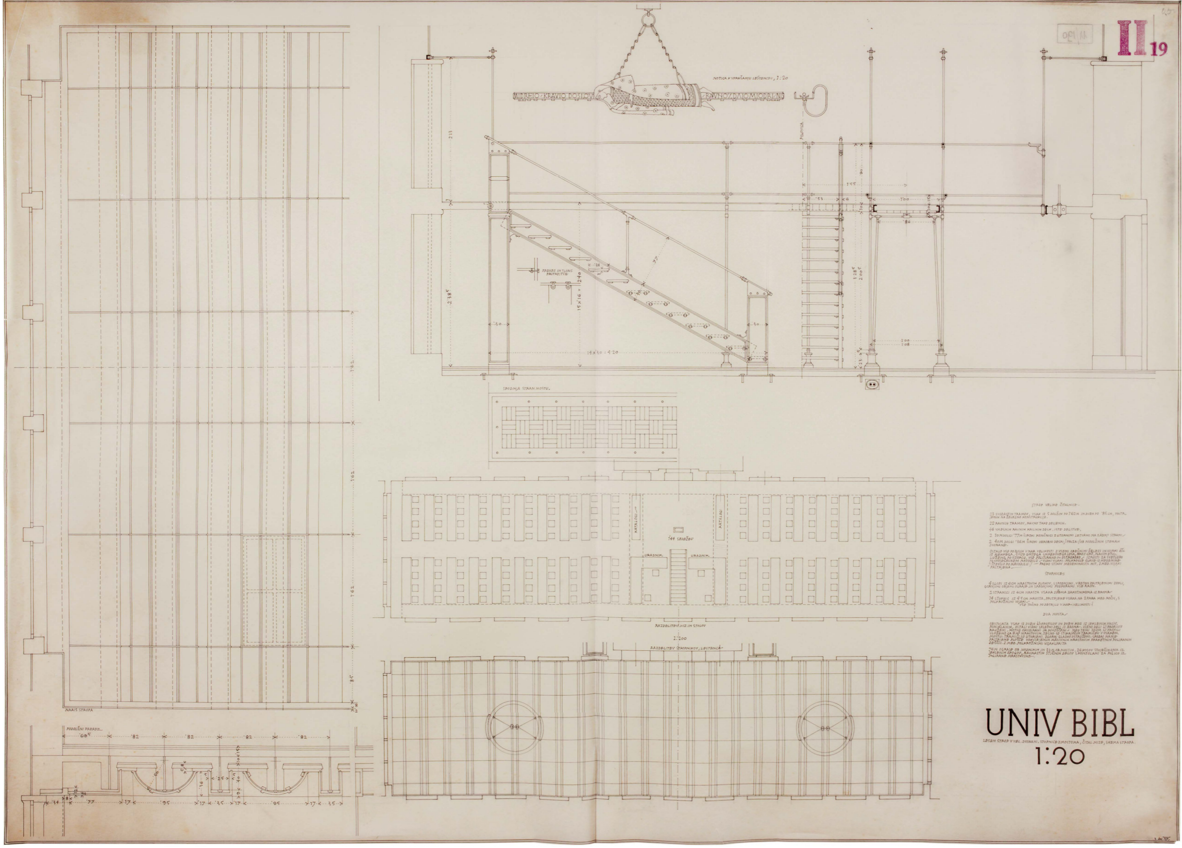
LXXX - Načrt čitalnice s stropom, pohištvom in mostovžem, 1:20, 3. 12. 1937
