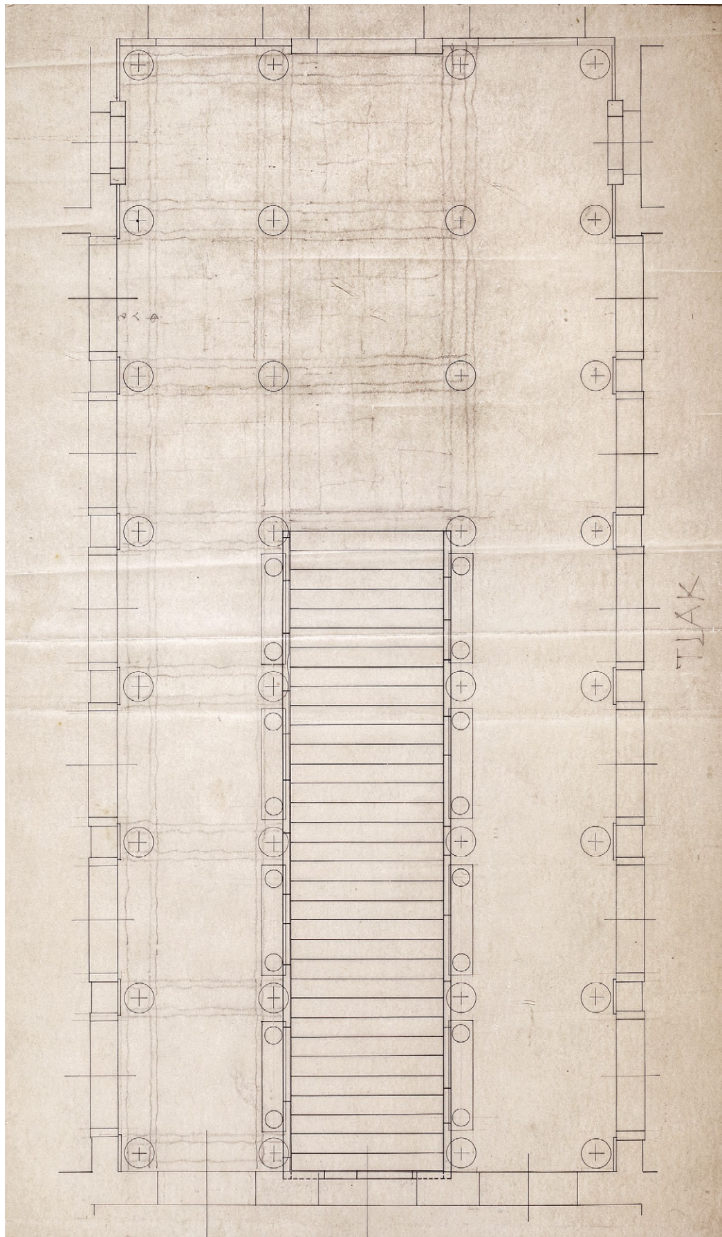
LXXII - Tloris peristila
