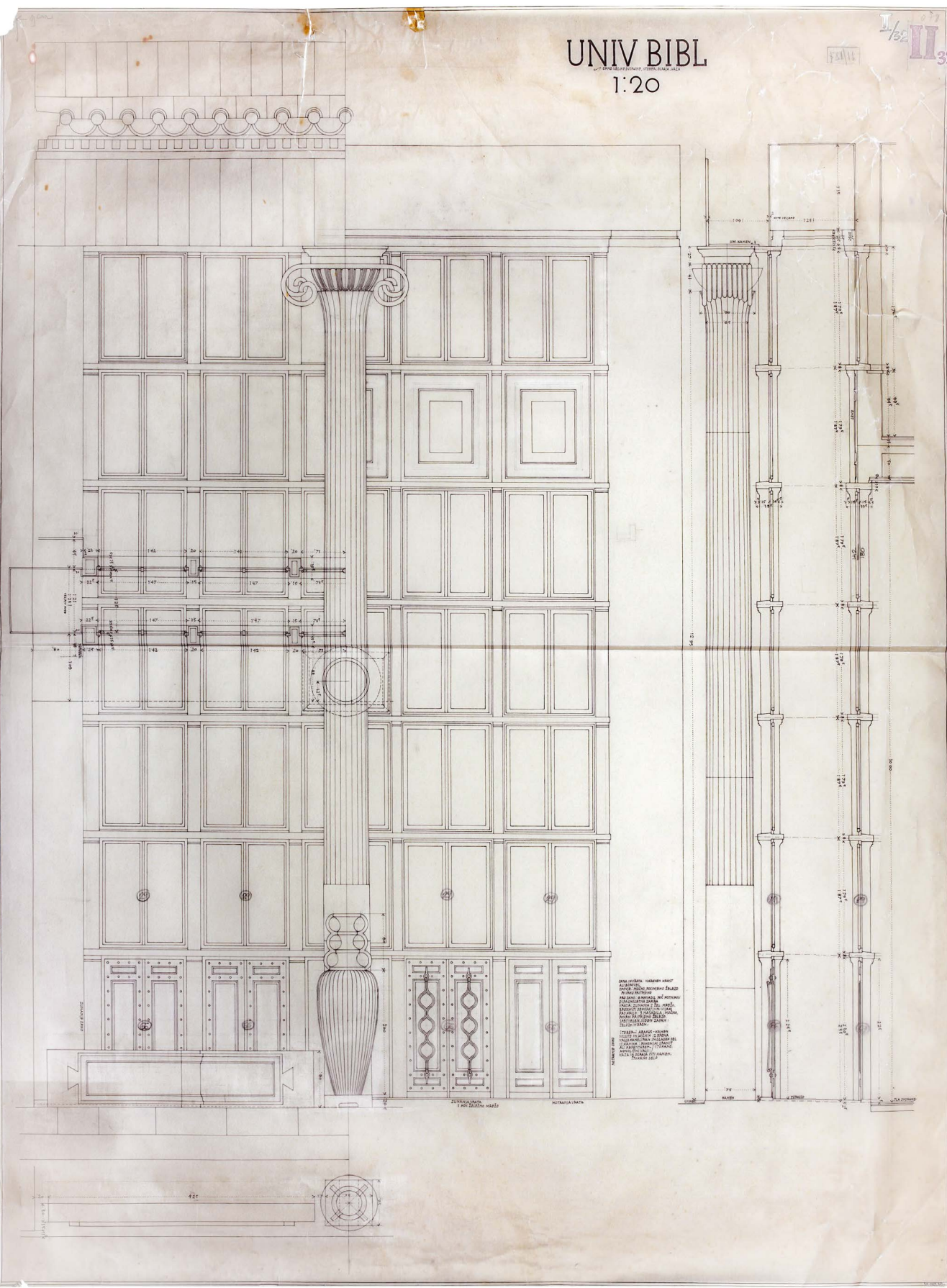
XLV - Načrt čitalniškega okna s stebrom in vazo, 1:20, 30. 10. 1937
