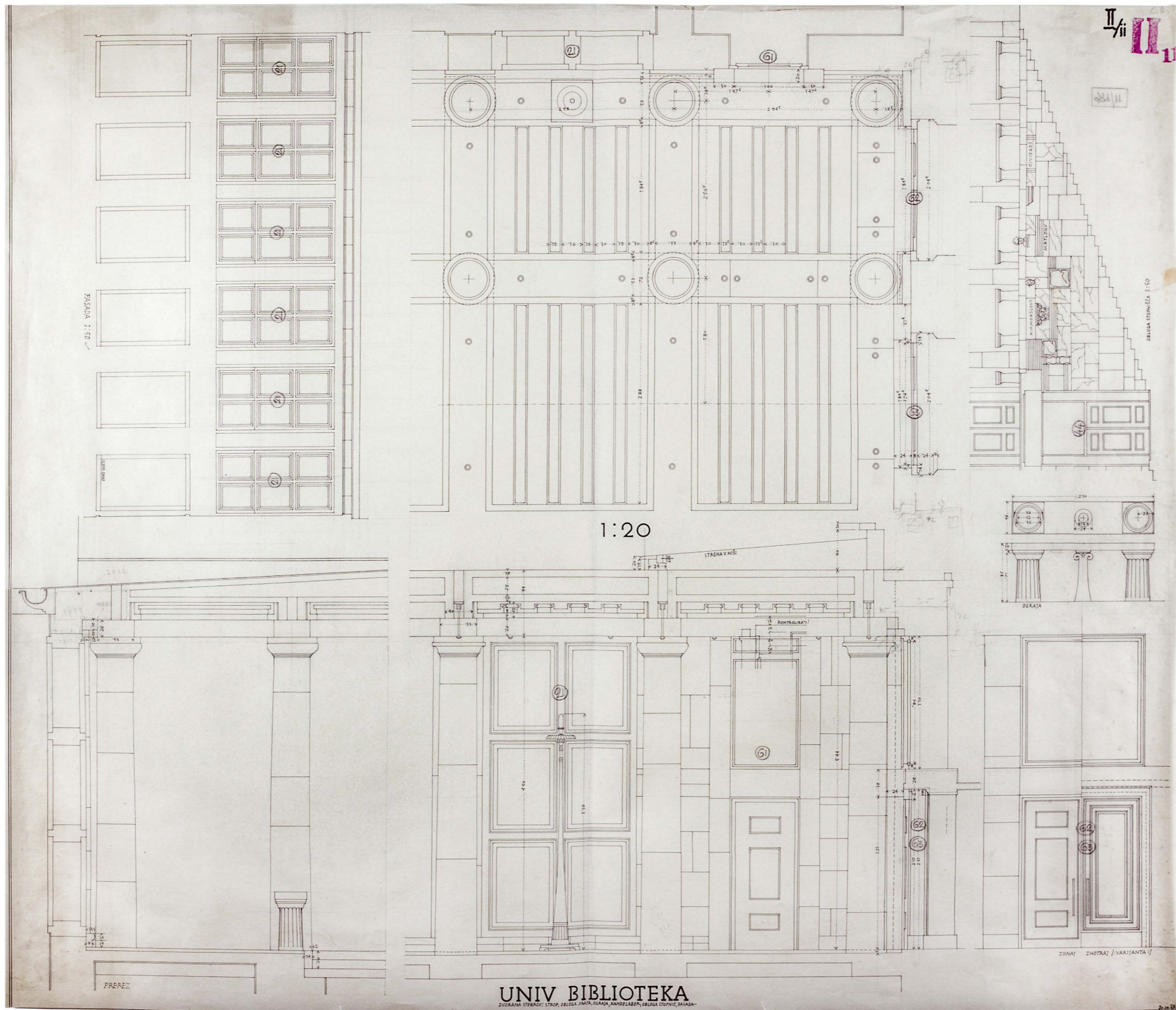
LV - Načrt peristila, 1:20, 20. 9. 1937
