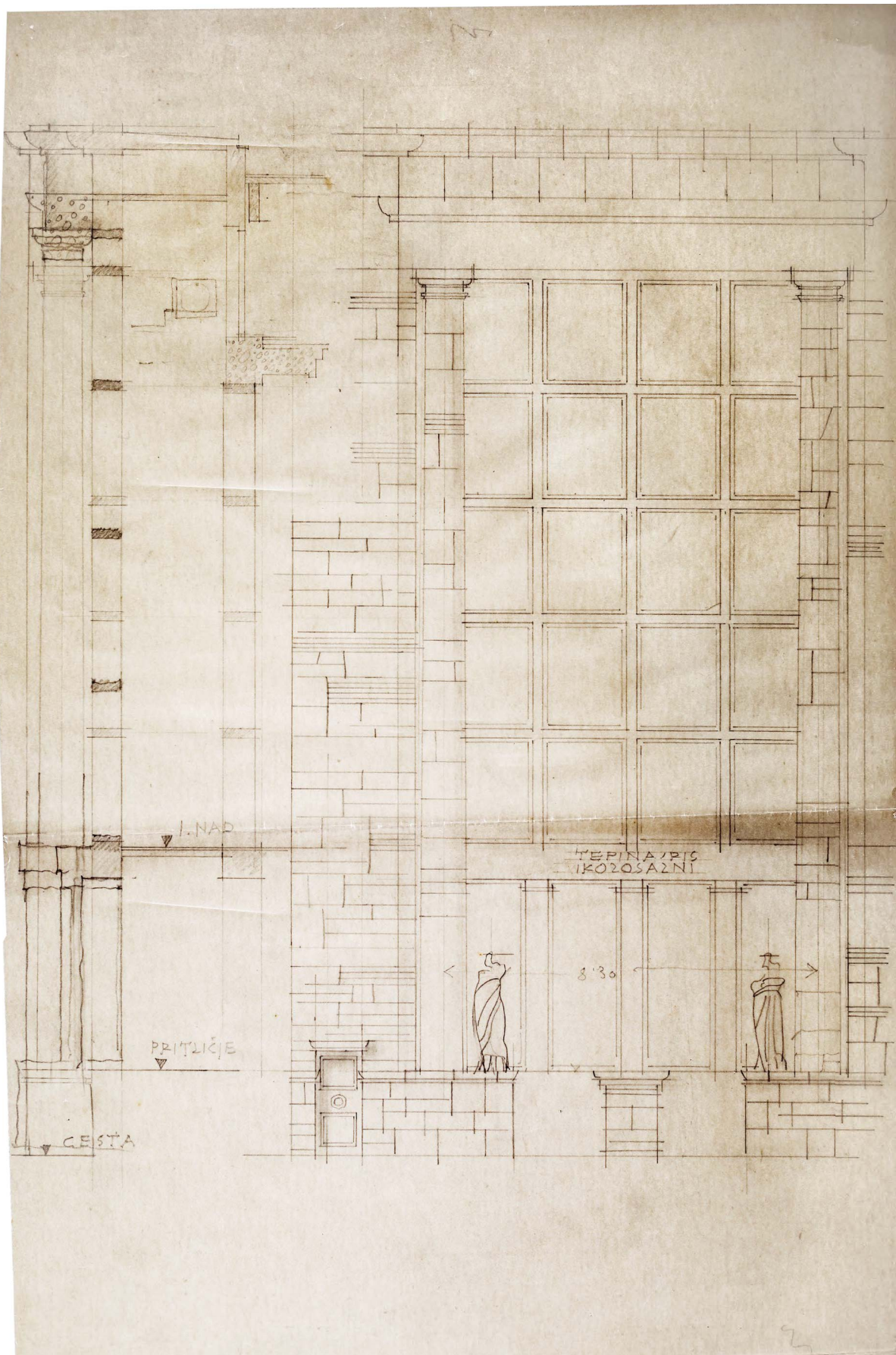
XLVII - Ravnikarjeva risba čitalniškega okna s stebroma, na katero je Plečnik narisal dva kipa
