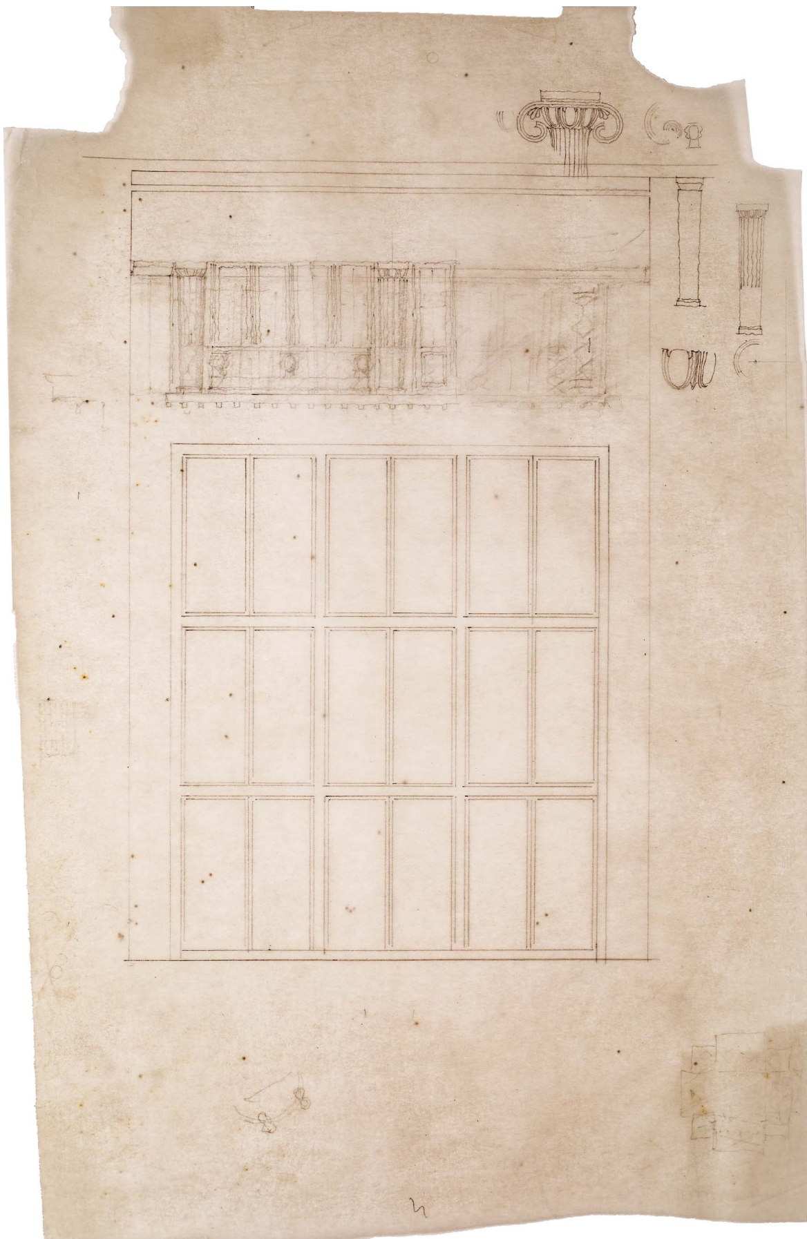
XLIX - Risba čitalniškega okna
