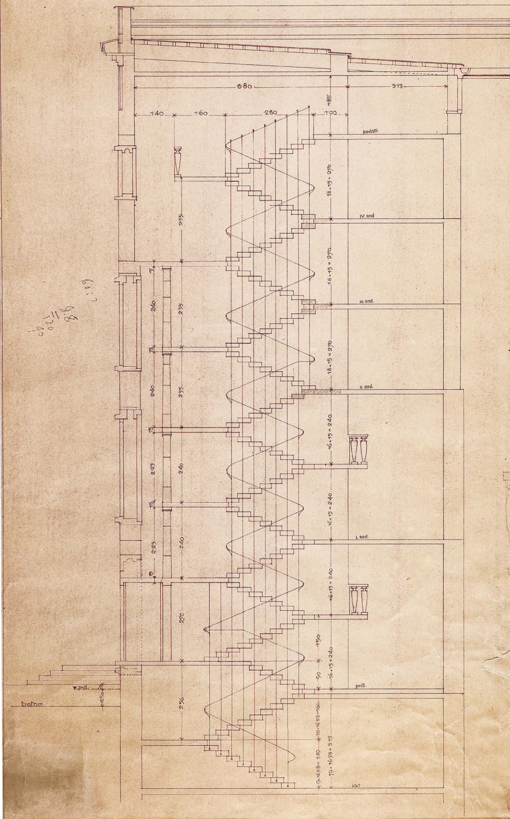
XC - Prerez stranskega stopnišča proti Vegovi ulici
