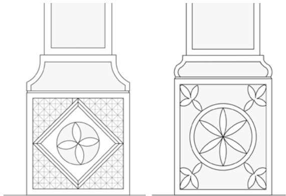
Zelo lepo okrašeni bazi dveh portalov pri Gorjupu v Lokovcu. Na risbah so robovi in drugi deli portala, ki so obdelani z dletom ali zglajeni, beli, hrupave ploskve, obdelane z zobatim kladivom ali krempačem, pa rahlo sivo osenčene. Risba Teje Mržek
