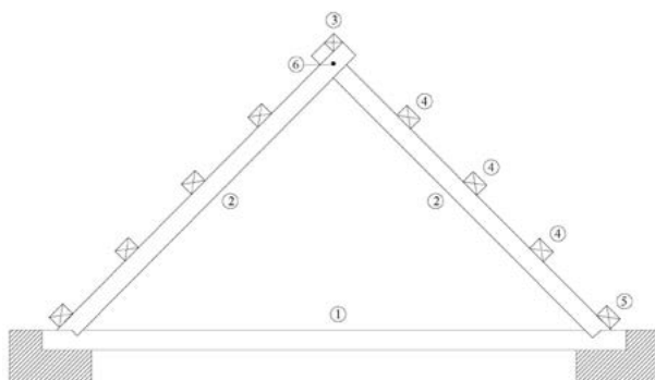
Škarjasto povezje z legami in slemenom na prekrížanih škarnikih: 1 – poveznik, 2 – škarnik, 3 – sleme, 4 – vmesne lege, 5 – kapna lega, 6 – lesen klin. Risba Teje Mržek
