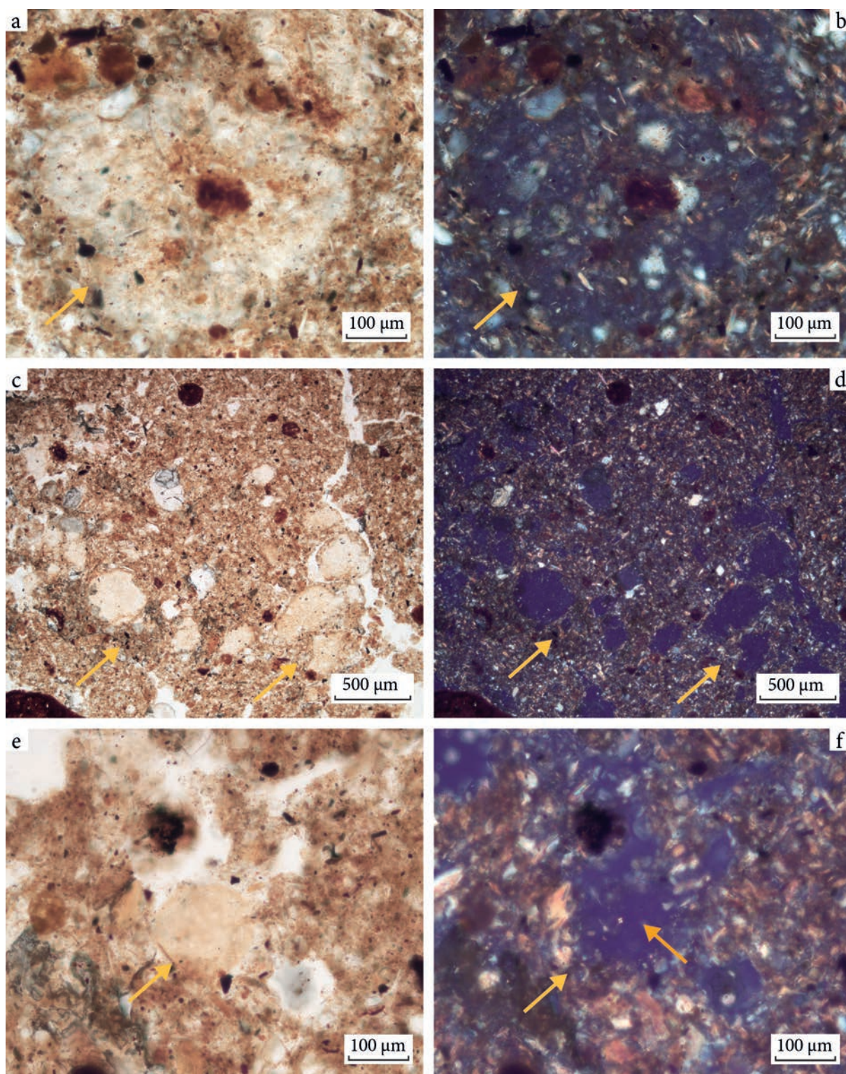
Sl. 8: Fosfatizirana amorfnna organska snov (a–d) in fosfatne nodule (e in f), vezane na mineralizacijo organske snovi v gnoju. V nekaterih fosfatnih nodulah (f, oranžna puščica) se pojavljajo posamični sferuliti (tj. sferično oblikovani kalcitni minerali, ki se tvorijo v črevesju drobnice in goveda; glej Canti, Brochier 2017). (a) in (b) horizont A2, profil tal P4; (c) in (d) horizont A2, profil tal P4; (e) in (f) horizont Bg1, profil tal P5. (a), (c) in (e): II nik; (b), (d) in (f): + nik.
