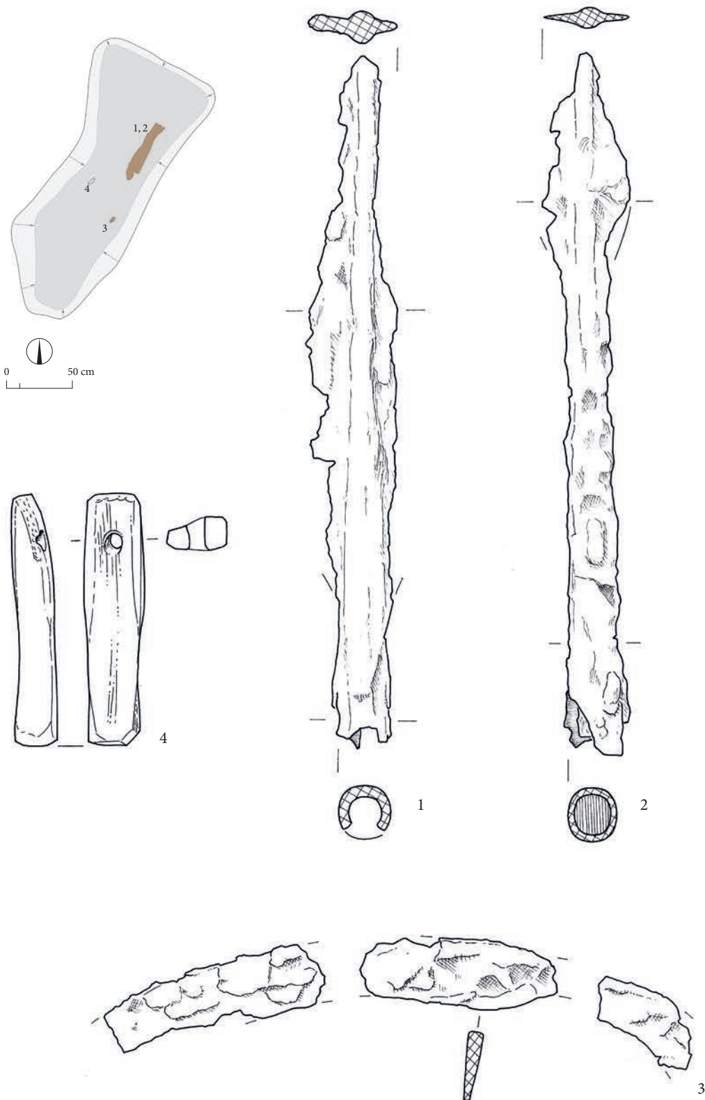
T. 28: Podzemelj, Pezdirčeva njiva: grob 70. 1–3 železo; 4 kamen. M. = 1:2.
