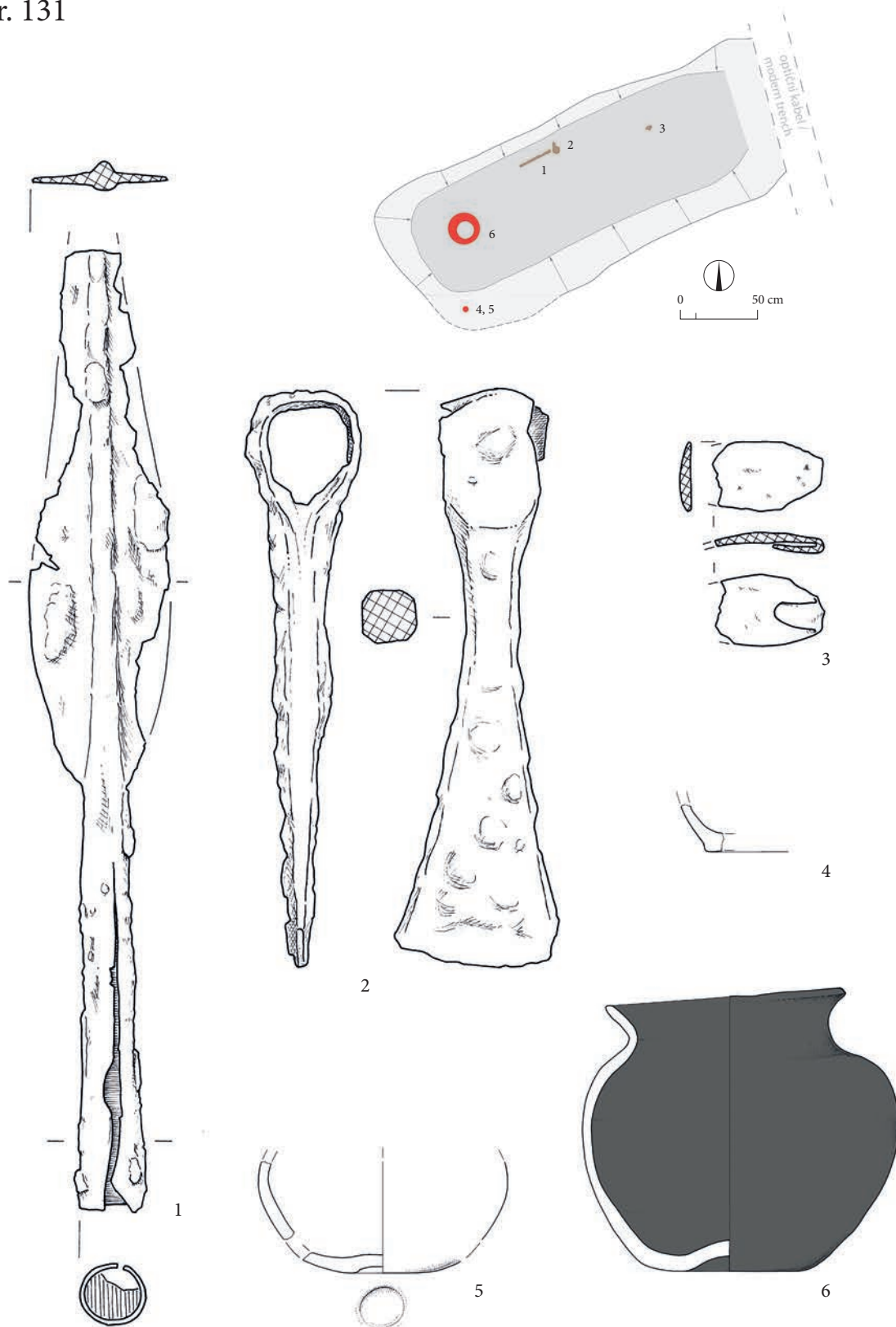
T. 64: Podzemelj, Pezdirčeva njiva: grob 131. 1–3 železo; 4–6 keramika. M. 1–3 = 1:2; ostalo = 1:4.
