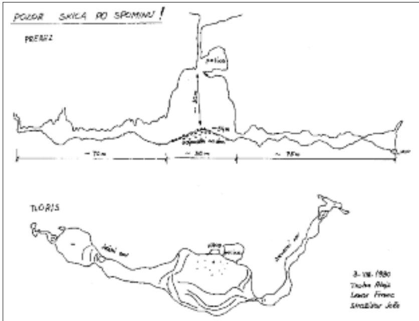
Slika 22: Tlorisni načrt Anžetove jame (Kataster jam JZS 2011).
