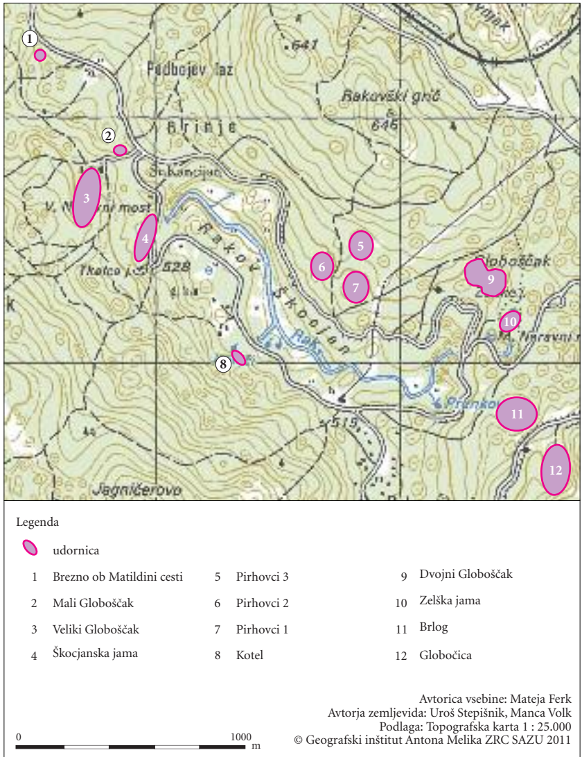
Slika 25: Lokacije udornic na območju Rakovega Škočjana.
