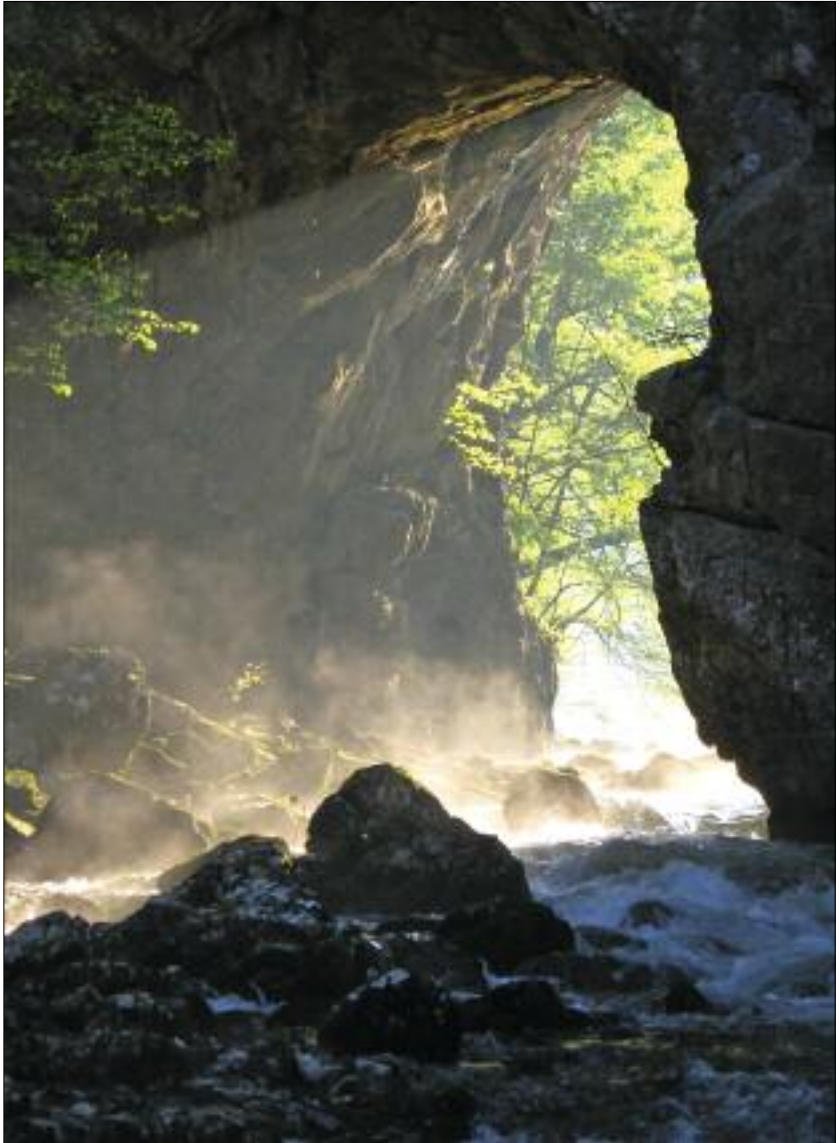
Slika 48: Veliki naravni most.
