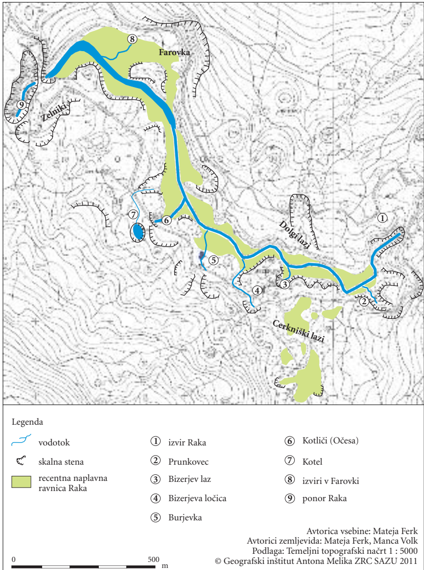
Slika 7: Geomorfološki zemljevid hidrološko aktivnega dna doline Raka.
